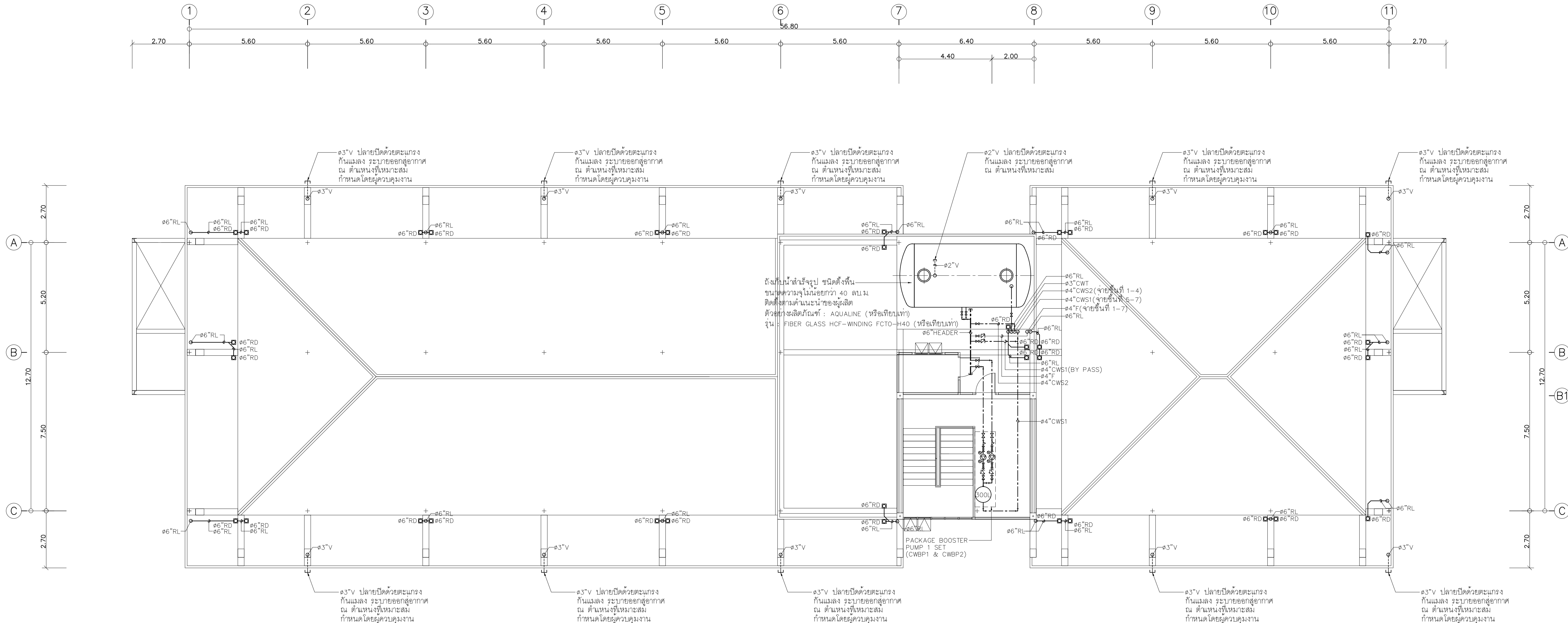
แผนระบบสุขภาพิบาลพื้นที่นหลังคา
