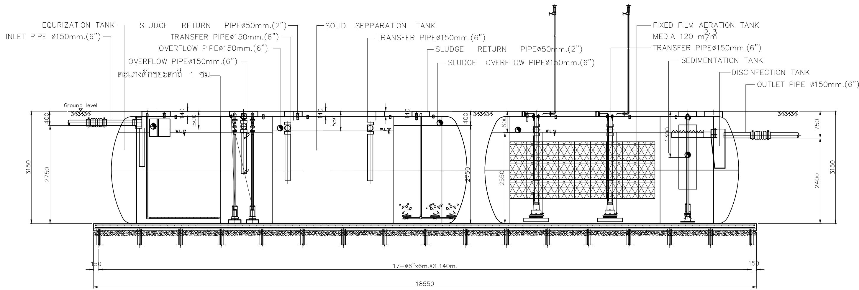
รูปตัด A-A ไม่แสดงขนาดบางส่วน
