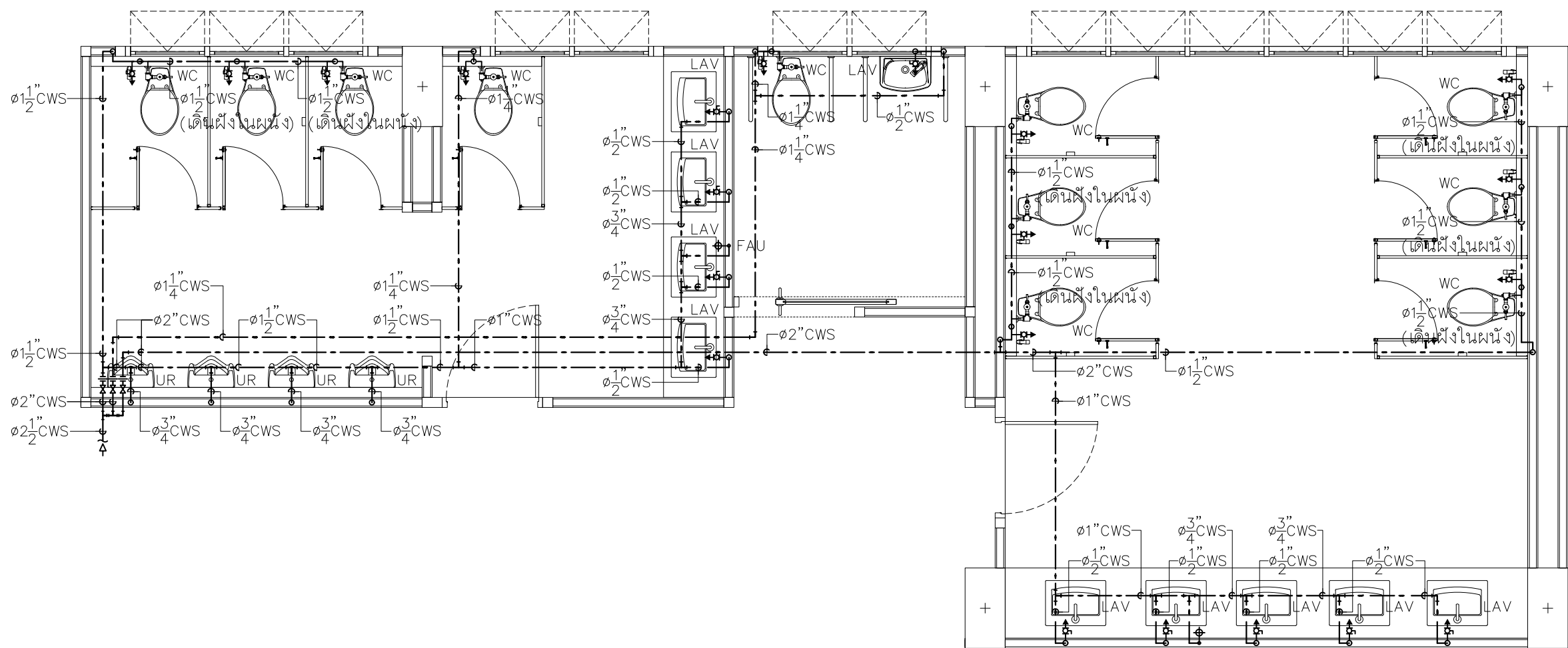
แบบขยายการเดินท่อ CWS ภายในห้องน้ำ T1
