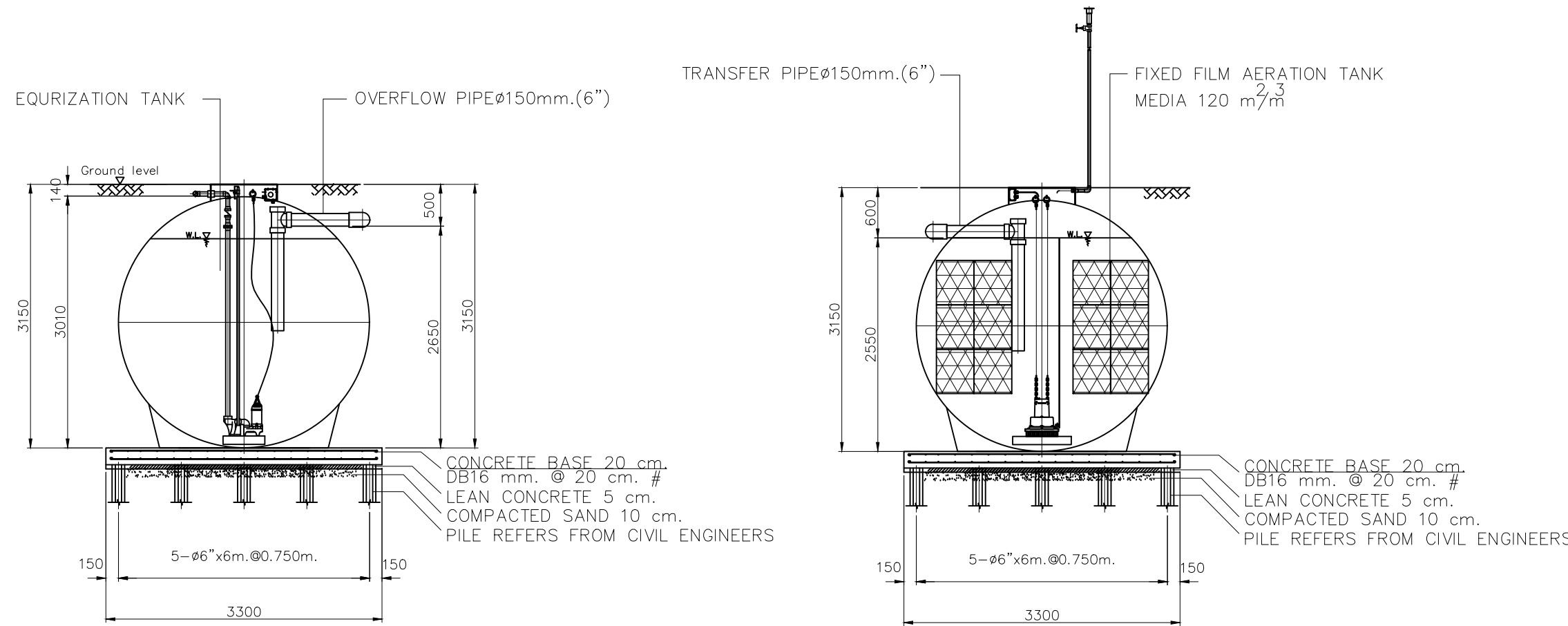
รูปตัด B-B ไม่แสดงขนาดบางส่วน
