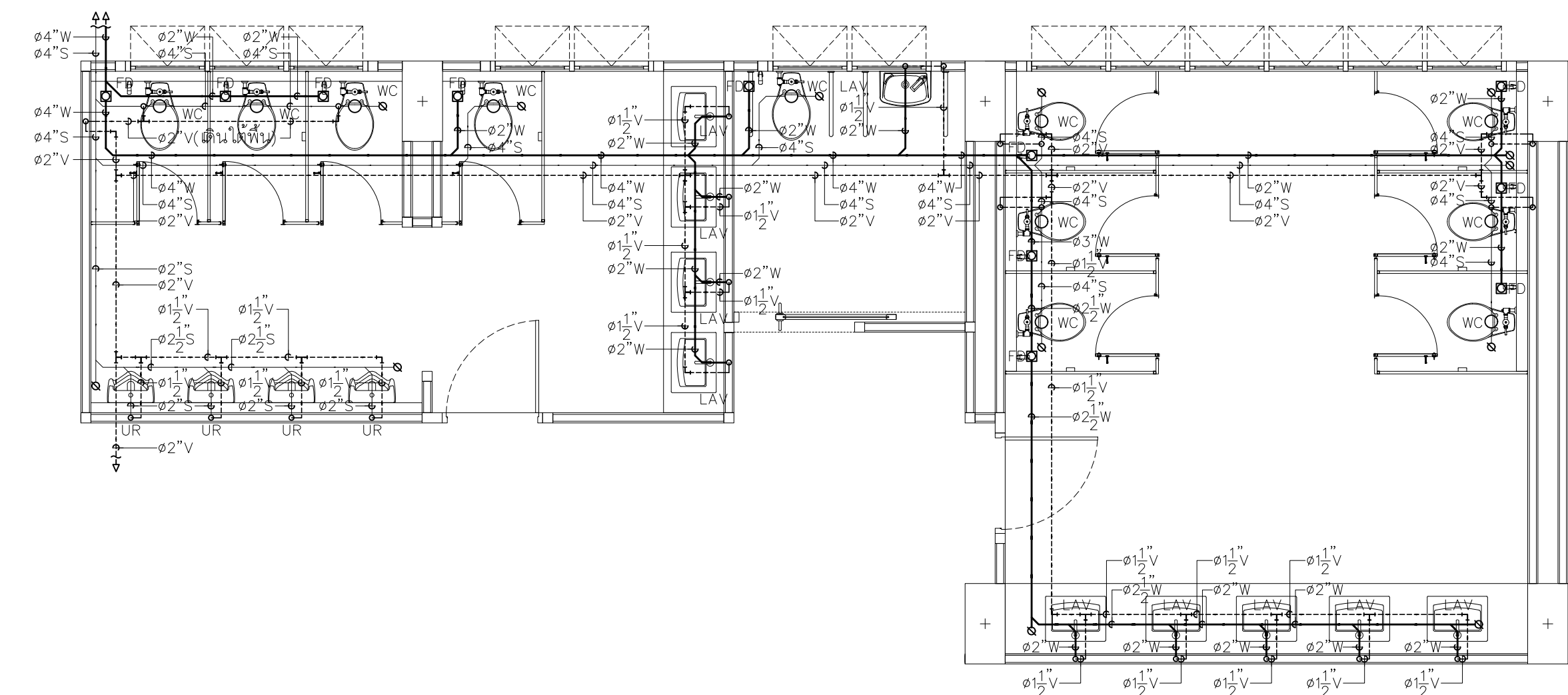
แบบขยายการเดินท่อ S,W,V ภายในห้องน้ำ T1
