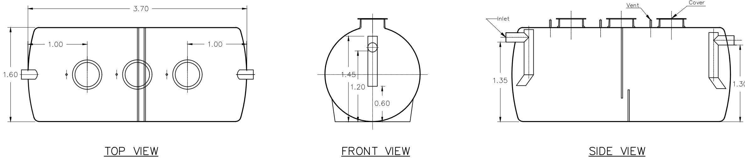
ถังตกไขมันสำหรับรูป ชนิดฝังดิน ขนาดความจุ 6 ลบ.ม. NOT TO SCALE
